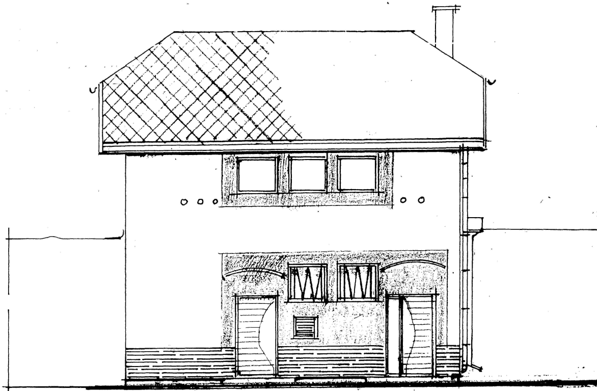
Elewacja północna 1:100
