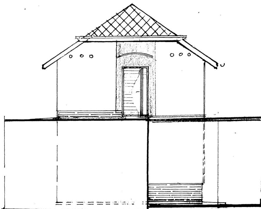
Elewacja wschodnia 1:100
